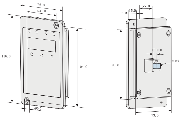
图8-16外引键盘的外型尺寸
