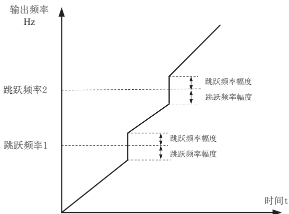
图6-18 加减速过程中跳跃频率有效示意图
