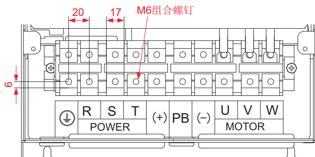
图8-6 SIZE E结构功率接线端子尺寸图
