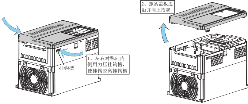
图3-12 塑胶外壳盖板拆卸图（FX8000）
