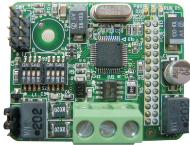
附录G：图1 FX8000CAN2外型
