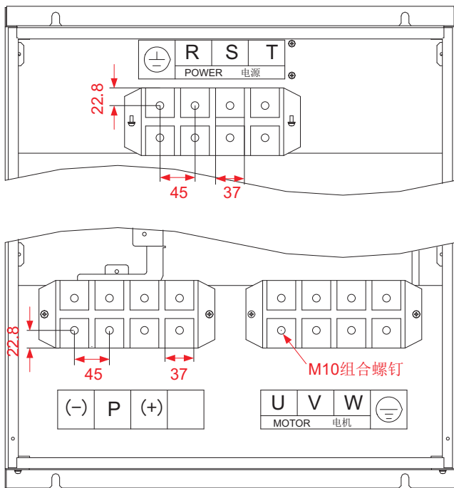
图8-9 SIZE H结构功率接线端子尺寸图
