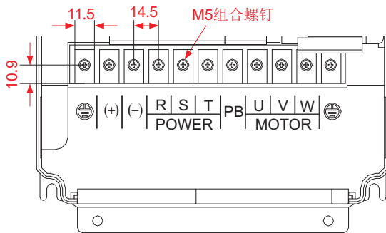
图8-5 SIZE D结构功率接线端子尺寸图
