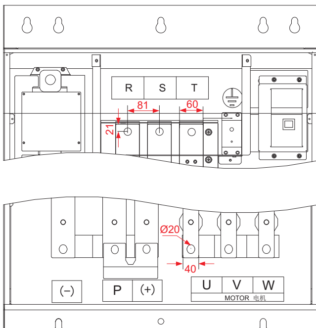
图8-11 SIZE J结构功率接线端子尺寸图
