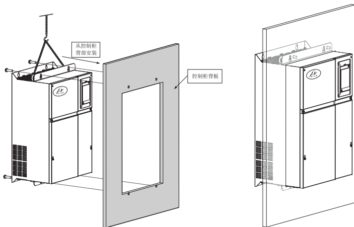
图3-10 塑胶结构嵌入式安装示意图
