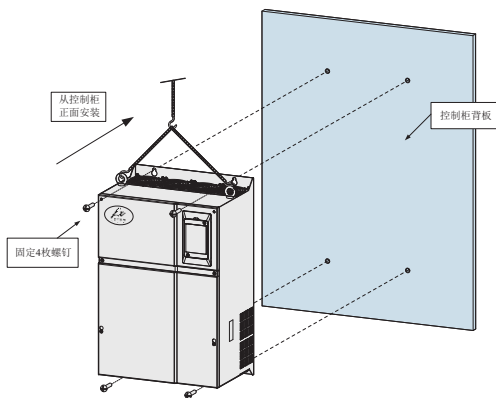
图3-7 钣金结构壁挂式安装示意图
