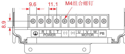
图8-4 SIZE C结构功率接线端子尺寸图
