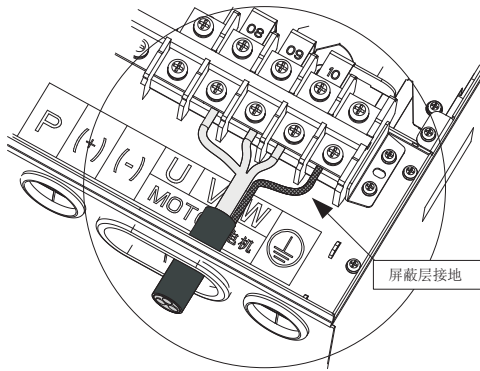
图7-1 屏蔽电缆接地示意图
