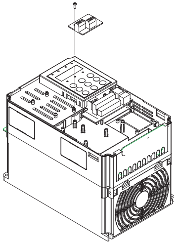
附录B：图1 FX8000IO2安装方式
