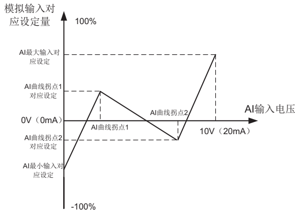
图6-33 曲线4和曲线5示意图
