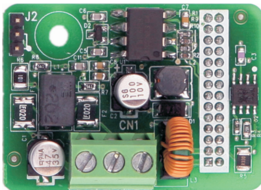
附录F：图1 FX8000CAN1外观
