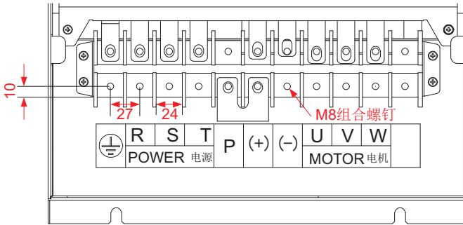
图8-7 SIZE F结构功率接线端子尺寸图
