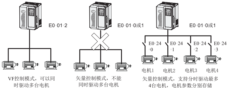
图4-29 多组电机的切换
