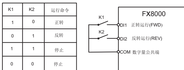
图6-6 两线式模式1
