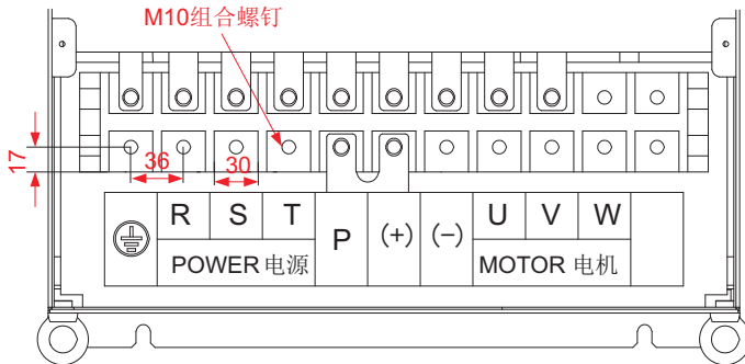
图8-8 SIZE G结构功率接线端子尺寸图
