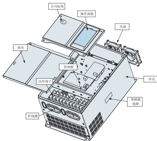
图2-3 FX8000系列变频器钣金结构外型图
