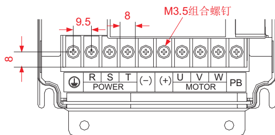
图8-3 SIZE B结构功率接线端子尺寸图
