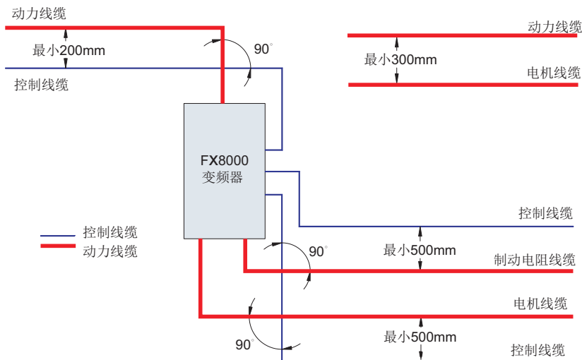
图7-2 电缆布线图
