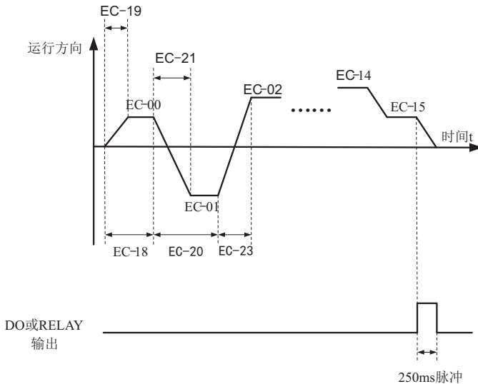
图6-31 简易PLC示意图
