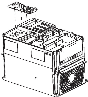
附录E：图 1 编码器扩展卡安装方式
