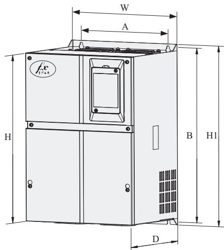
图8-2 FX8000系列 钣金结构外型尺寸及安装尺寸示意图
