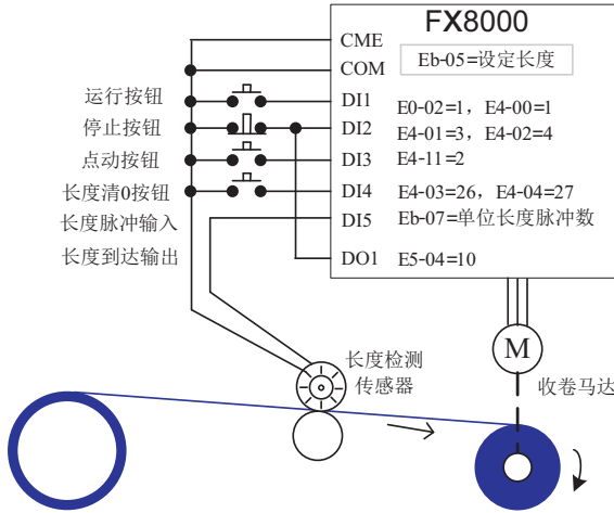
图4-27 定长控制功能常见应用举例
