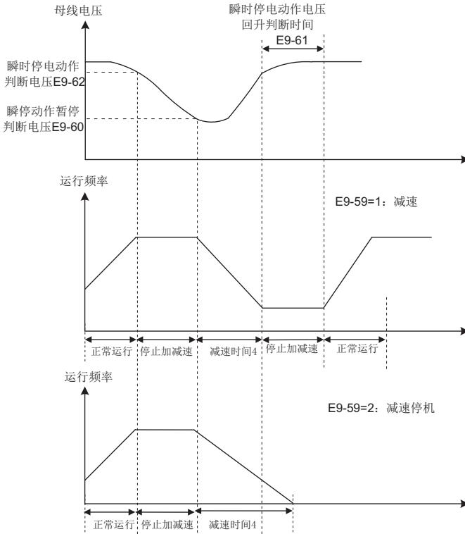
图6-25 瞬时停电动作示意图
