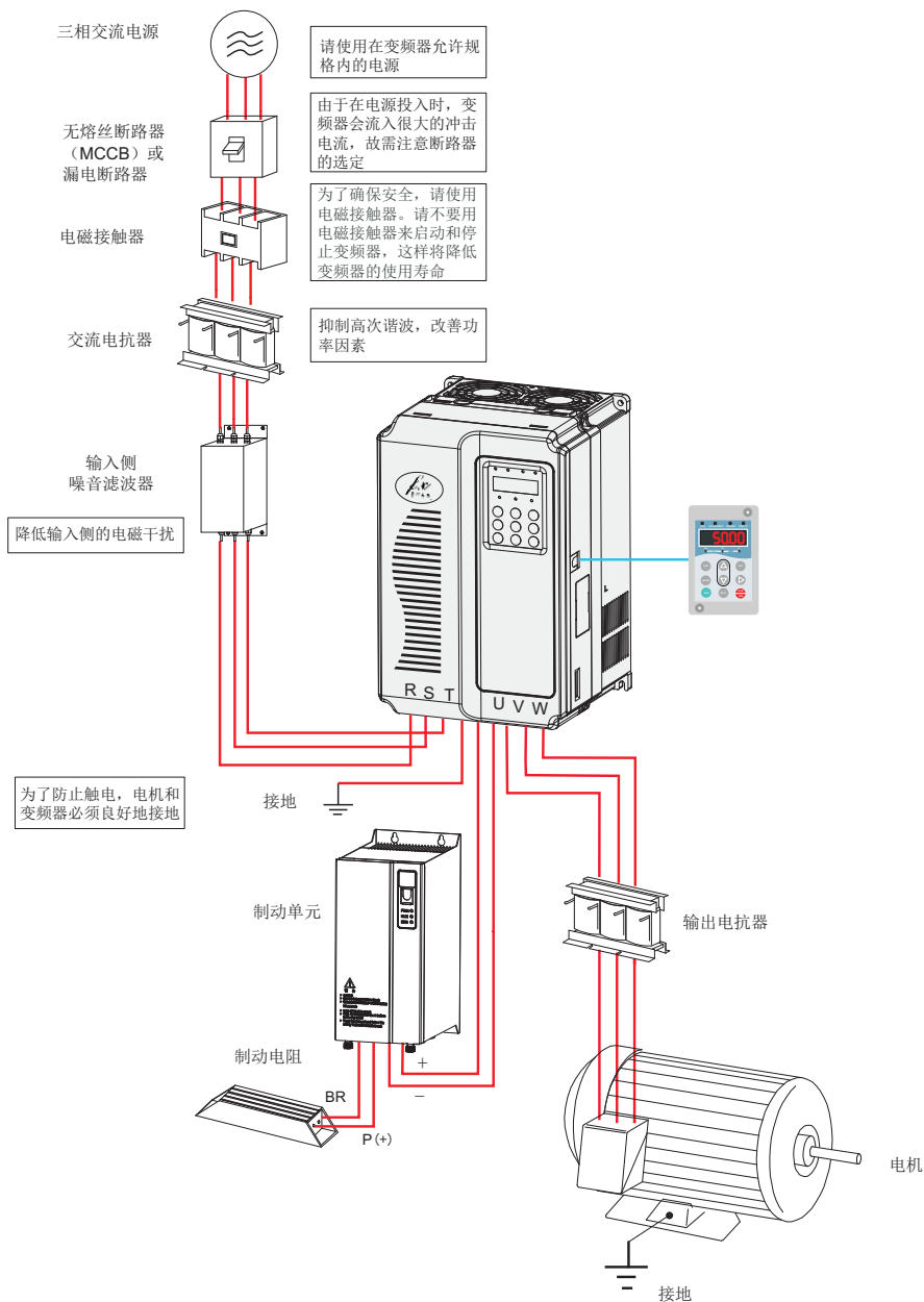
图2-4 380V系列系统构成
