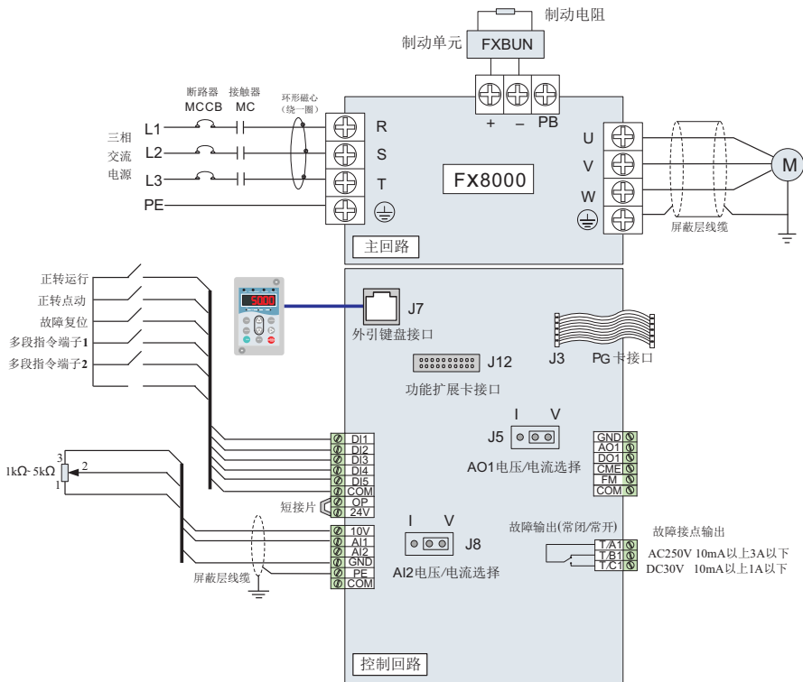
图3-22 FX8000电气接线示例
