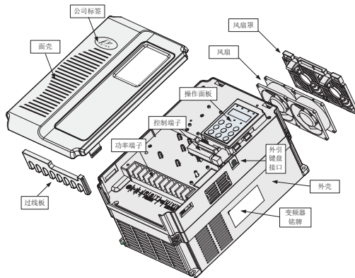
图2-2 FX8000系列变频器塑胶结构外型图
