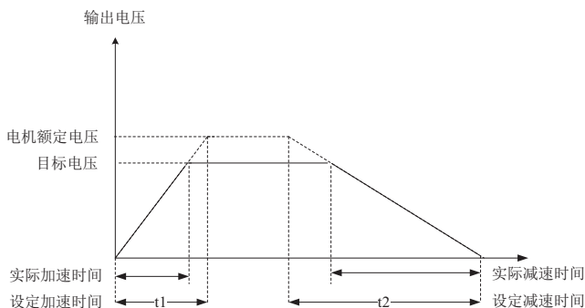
图6-5 V/F分离示意图
