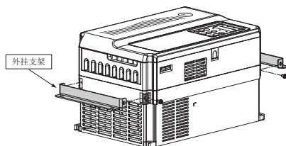
图3-4 塑胶结构安装外挂支架示意图
