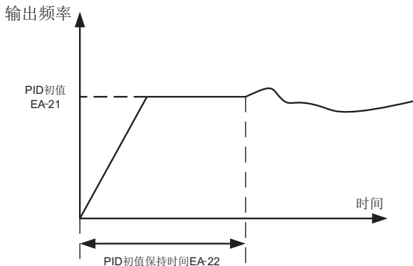
图6-28 PID初值功能示意图
