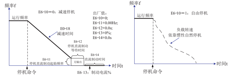
图4-11 停机模式
