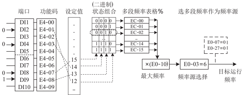
图4-24 多段速模式的设置
