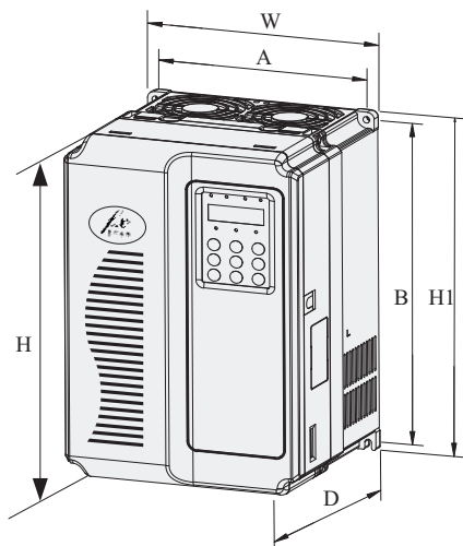
图8-1 FX8000系列 塑胶结构外型尺寸及安装尺寸示意图
