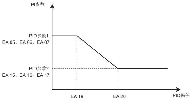
图6-27 PID参数切换
