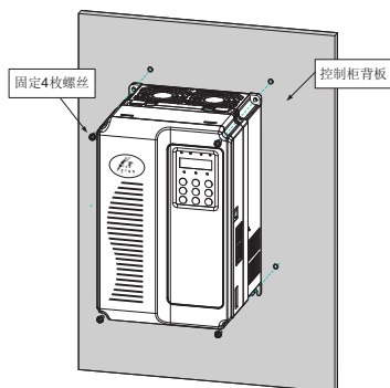
图3-3 塑胶结构壁挂式安装示意图
