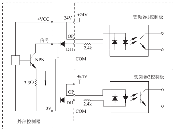
图3-19 多台变频器DI端子并联漏型接线方式
