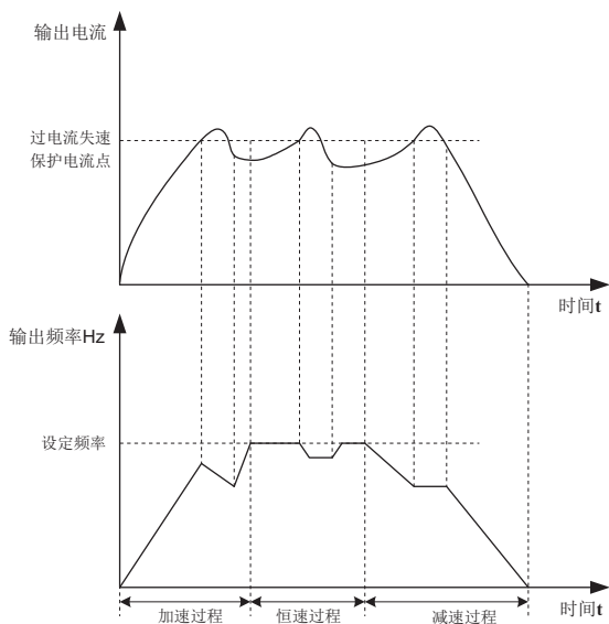
图6-24 过流失速保护示意图
