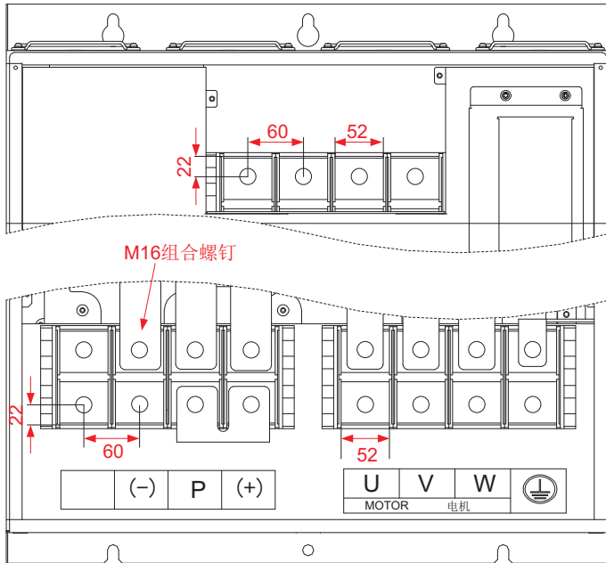
图8-10 SIZE I结构功率接线端子尺寸图
