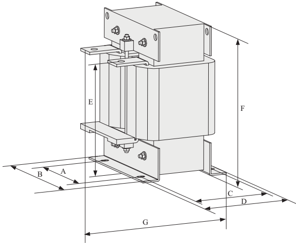
图8-15 外置电抗器尺寸示意图
